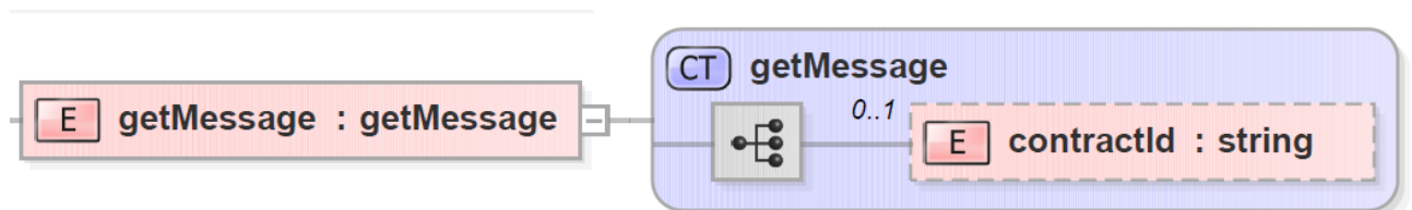
16. ábra: A getMessage adatsomag szerkezete
