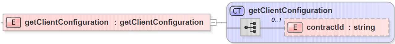
1. ábra: getClientConfiguration adatcsomagjának szerkezete
