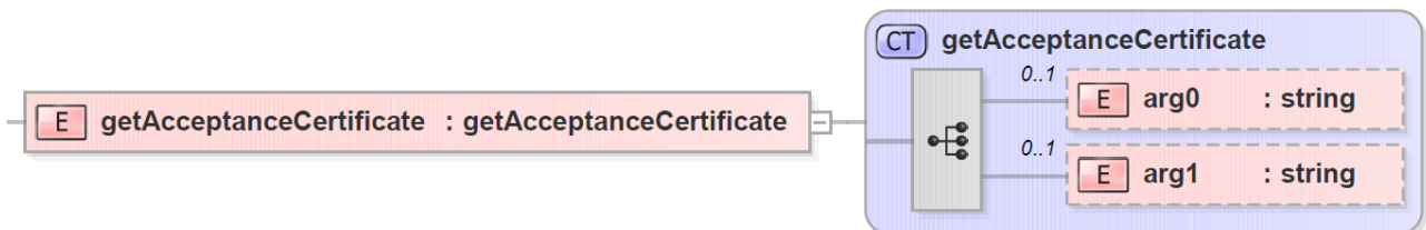
20. ábra: A getAcceptanceCertificate adatcsomagjának szerkezete
